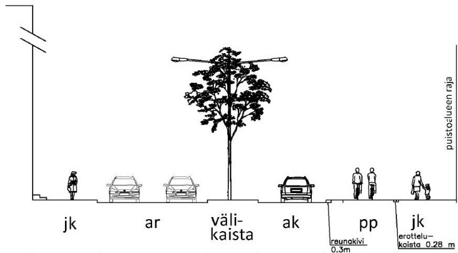
Ote Rautatienkadun alustavan yleissuunnitelman luonnoksesta. Katupoikkileikkaus Posteljoonipuiston kohdalla. (lähde: Tampereen kaupunki ja Ramboll Finland Oy 2020)
